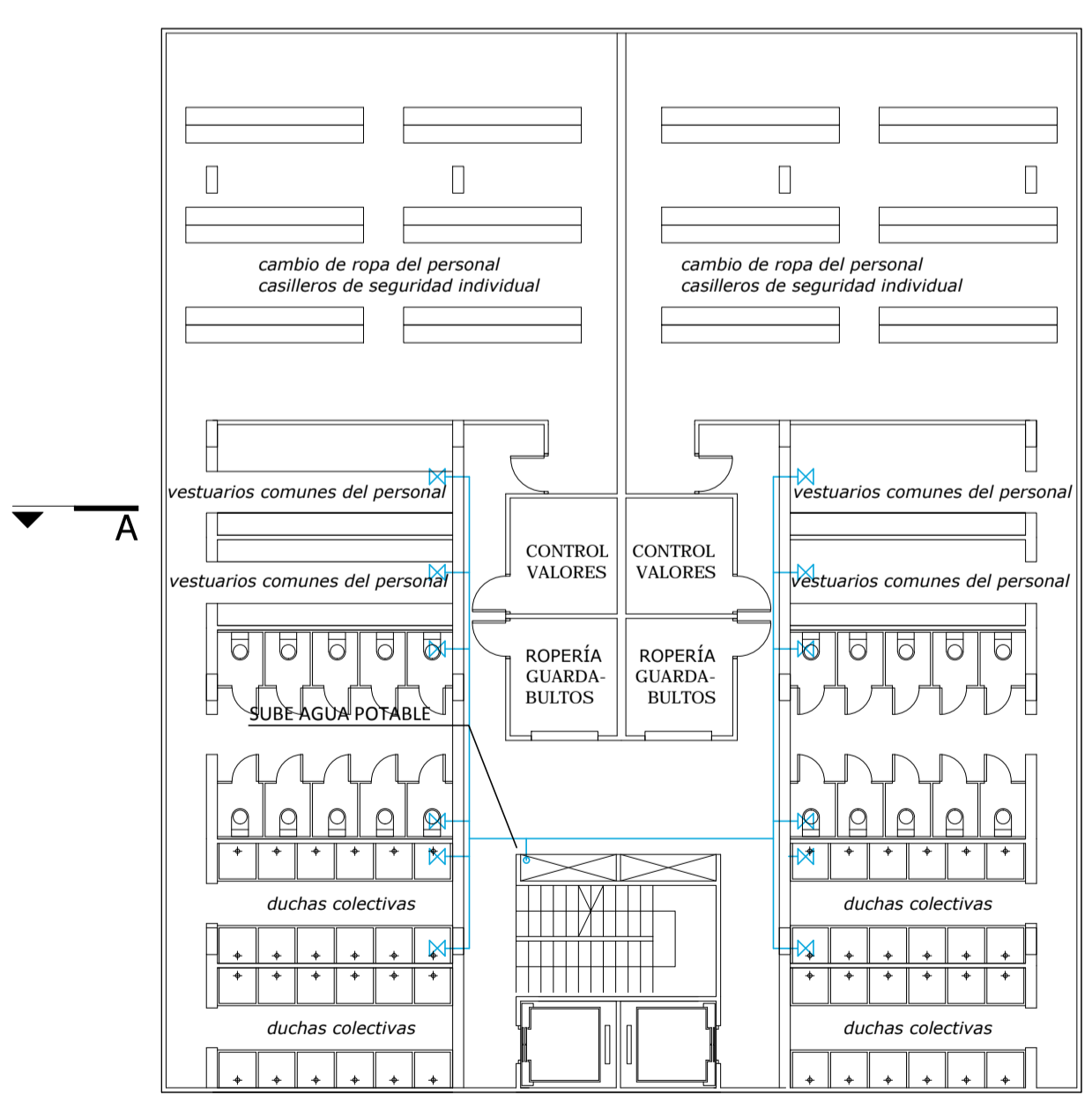
PISO 1 ESCALA: 1:250
