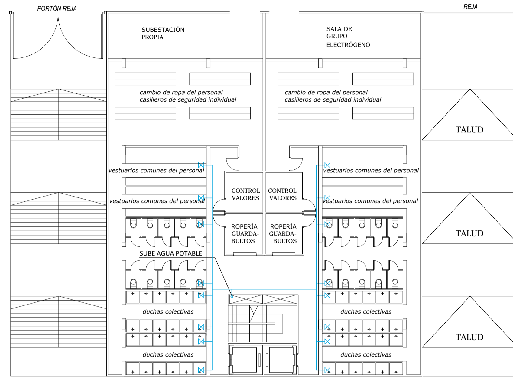
PLANTA BAJA ESCALA: 1:200
