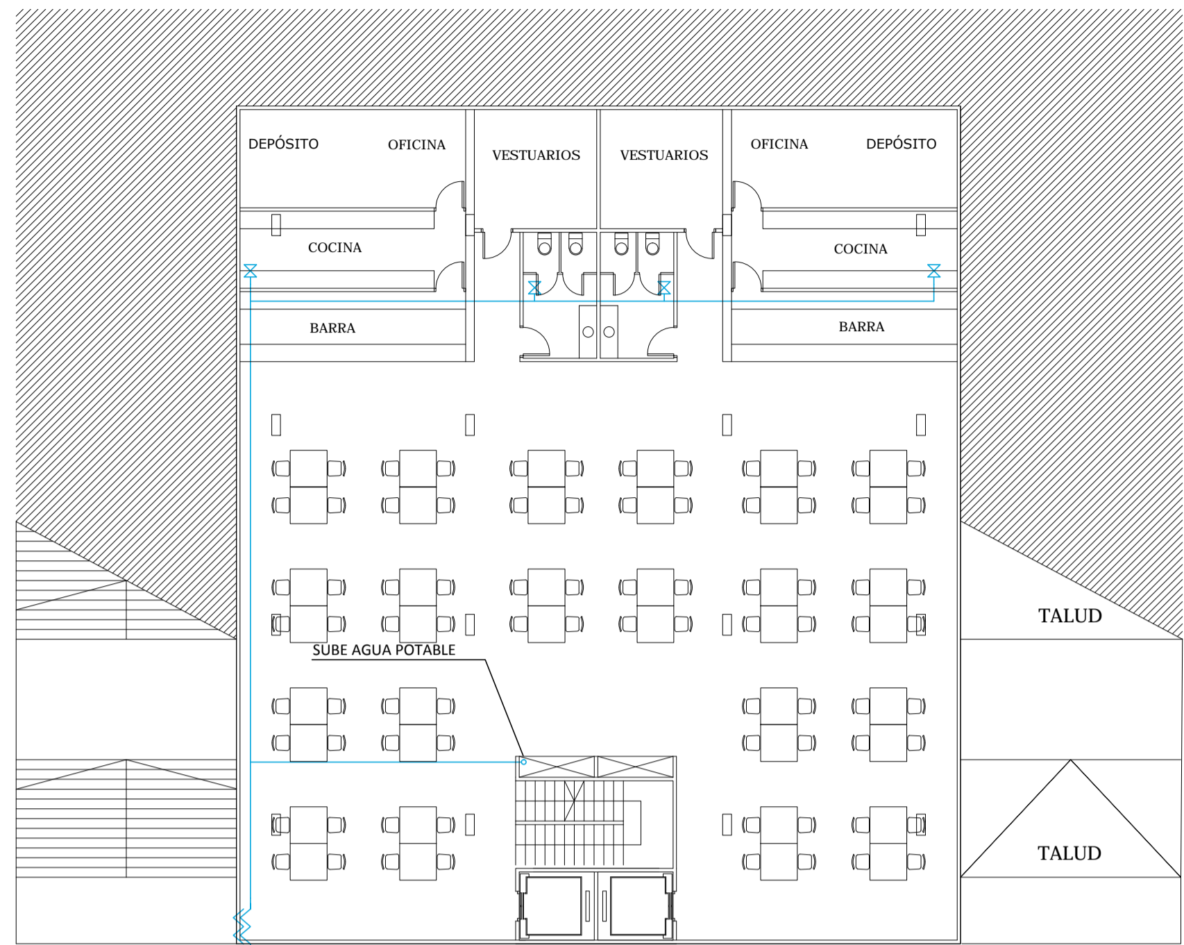
SUBSUELO 2 ESCALA: 1:200
