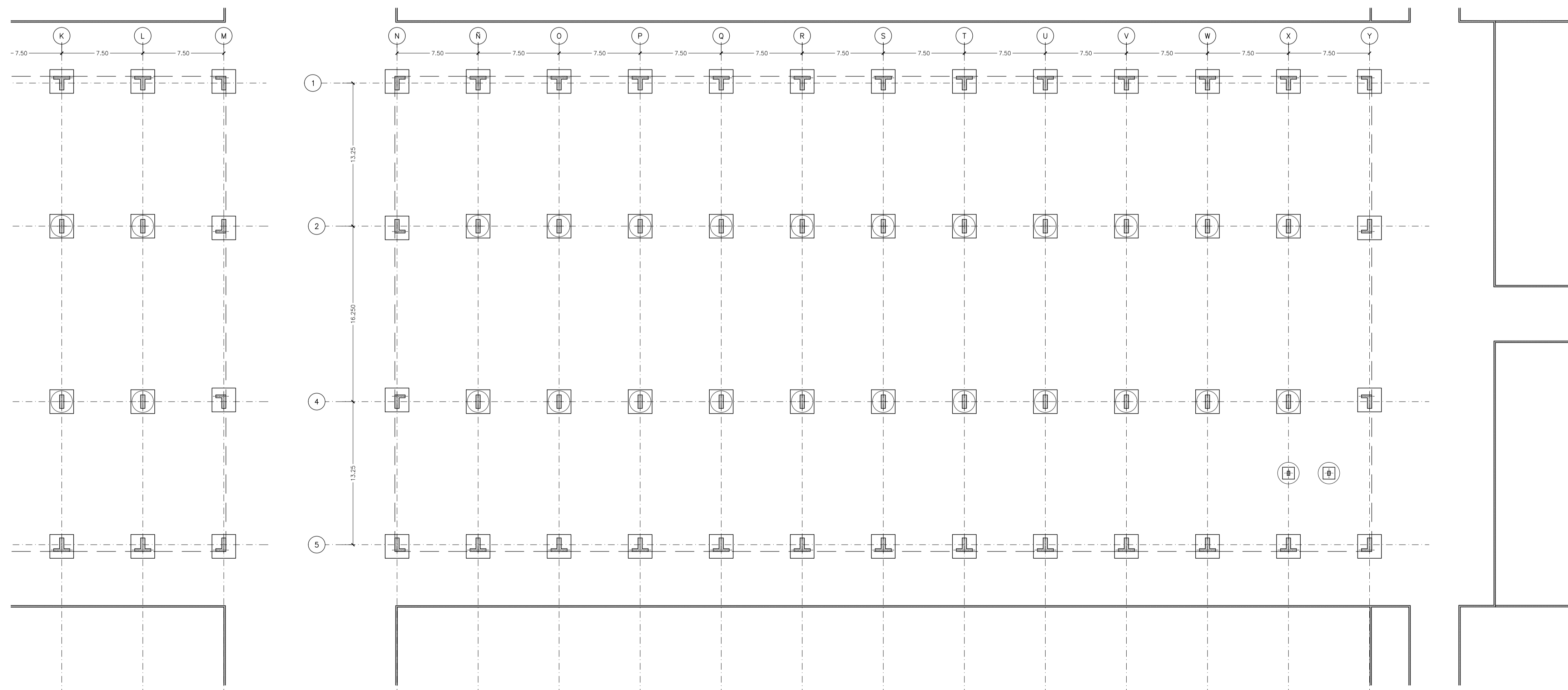
PLANTA ESQUEMATICA FUNDACIONES (VARIANTE FUNDACION DIRECTA) - ZONA B - ESC 1:250
