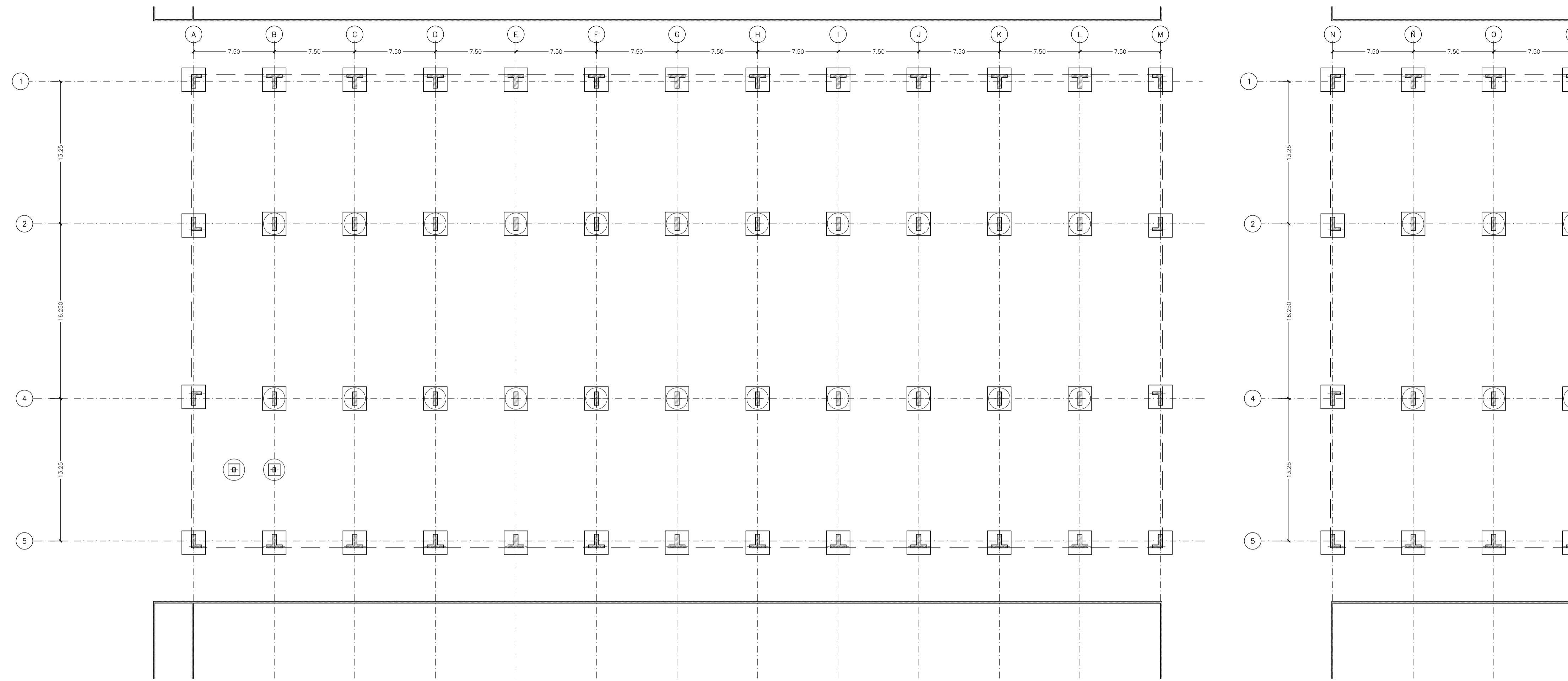
PLANTA ESQUEMATICA FUNDACIONES (VARIANTE FUNDACION DIRECTA) - ZONA A - ESC 1:250
