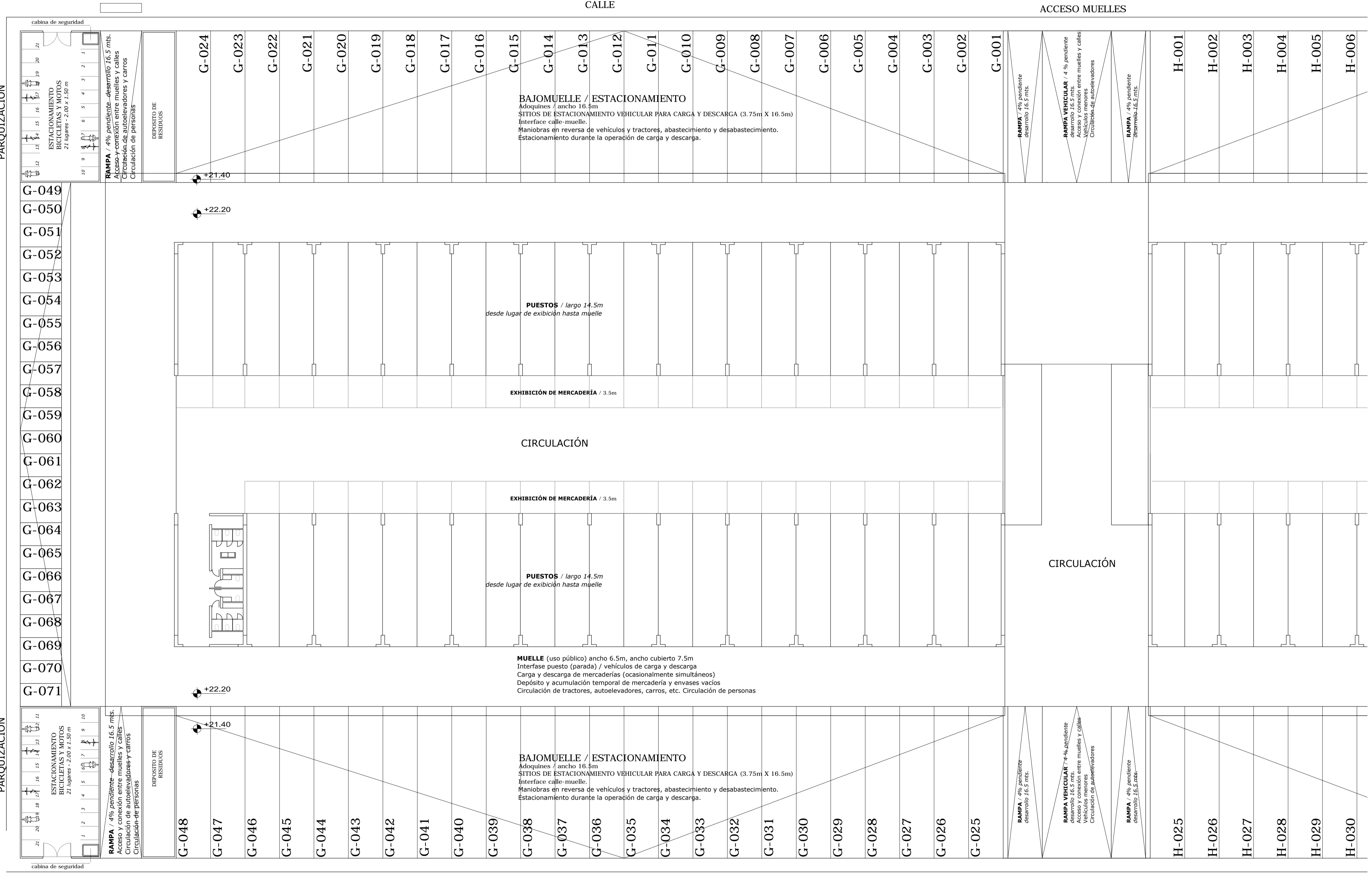
PLANTA PP (Sector Oeste) - ESC 1:250
