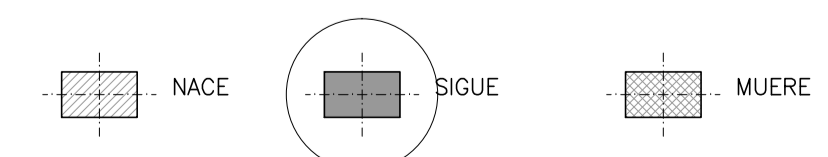
PLANTA ESQUEMATICA FUNDACIONES (VARIANTE PILOTES) - ESC 1:200
